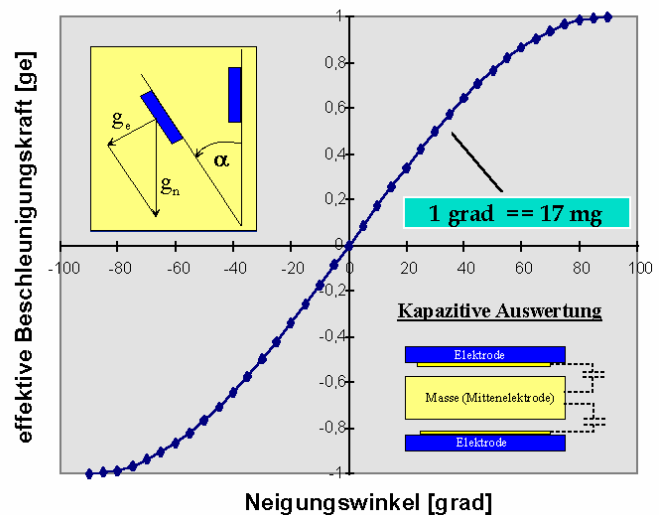
Effektive Beschleunigung in Abhängigkeit vom Neigungswinkel
